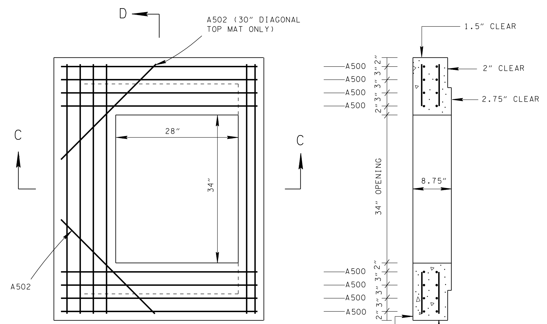
SECTION D-D
